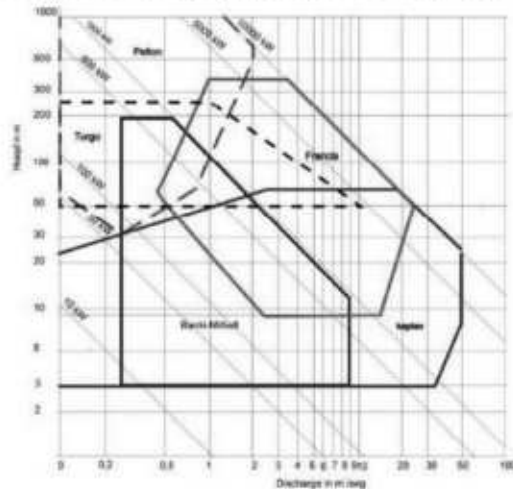
Gambar 14. Grafik Pemilihan Turbin
