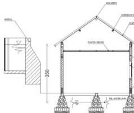
Gambar 12. Sketsa Tinggi Jatuh
