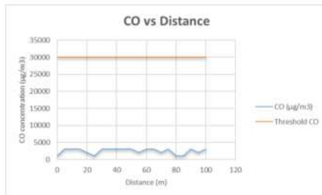
Gambar 6. Grafik Pengukuran Konsentrasi CO Terhadap Jarak
