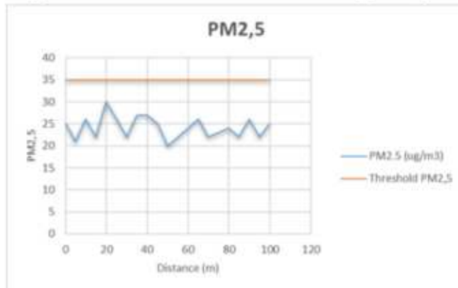
Gambar 5. Grafik Pengukuran Konsentrasi PM 2,5 Terhadap Jarak
