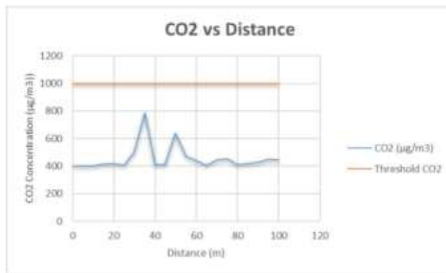
Gambar 7. Grafik Pengukuran Konsentrasi CO 2 Terhadap Jarak.
